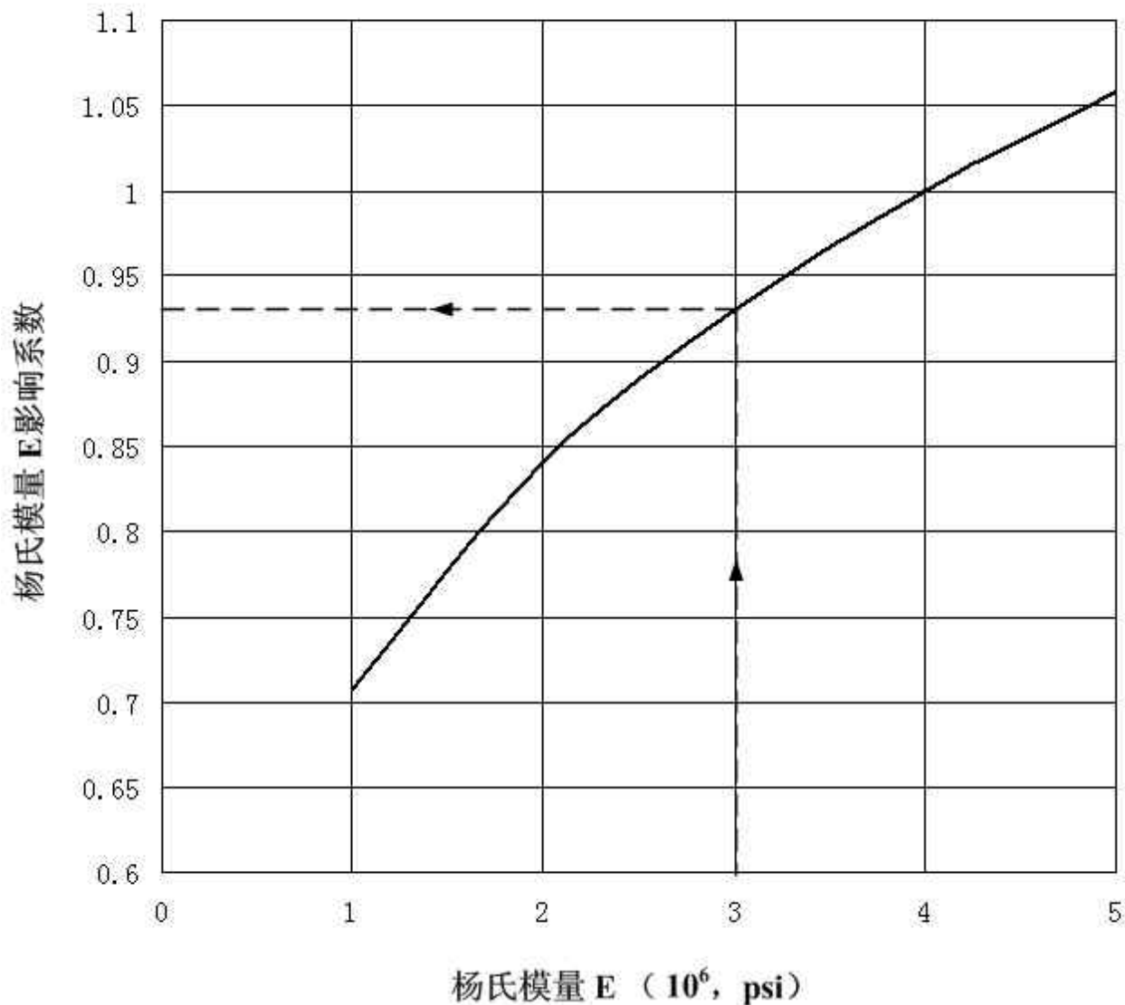
杨氏模量 E 对相对刚度半径 L 的影响
