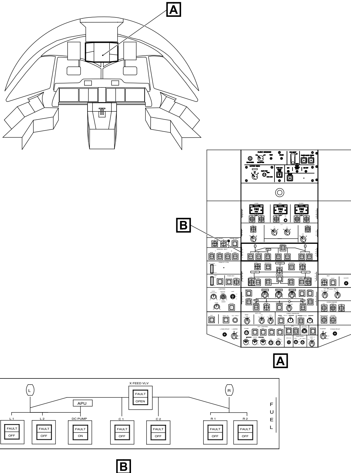
图 2 燃油 - 吸力放油 (共1张 第1张)
