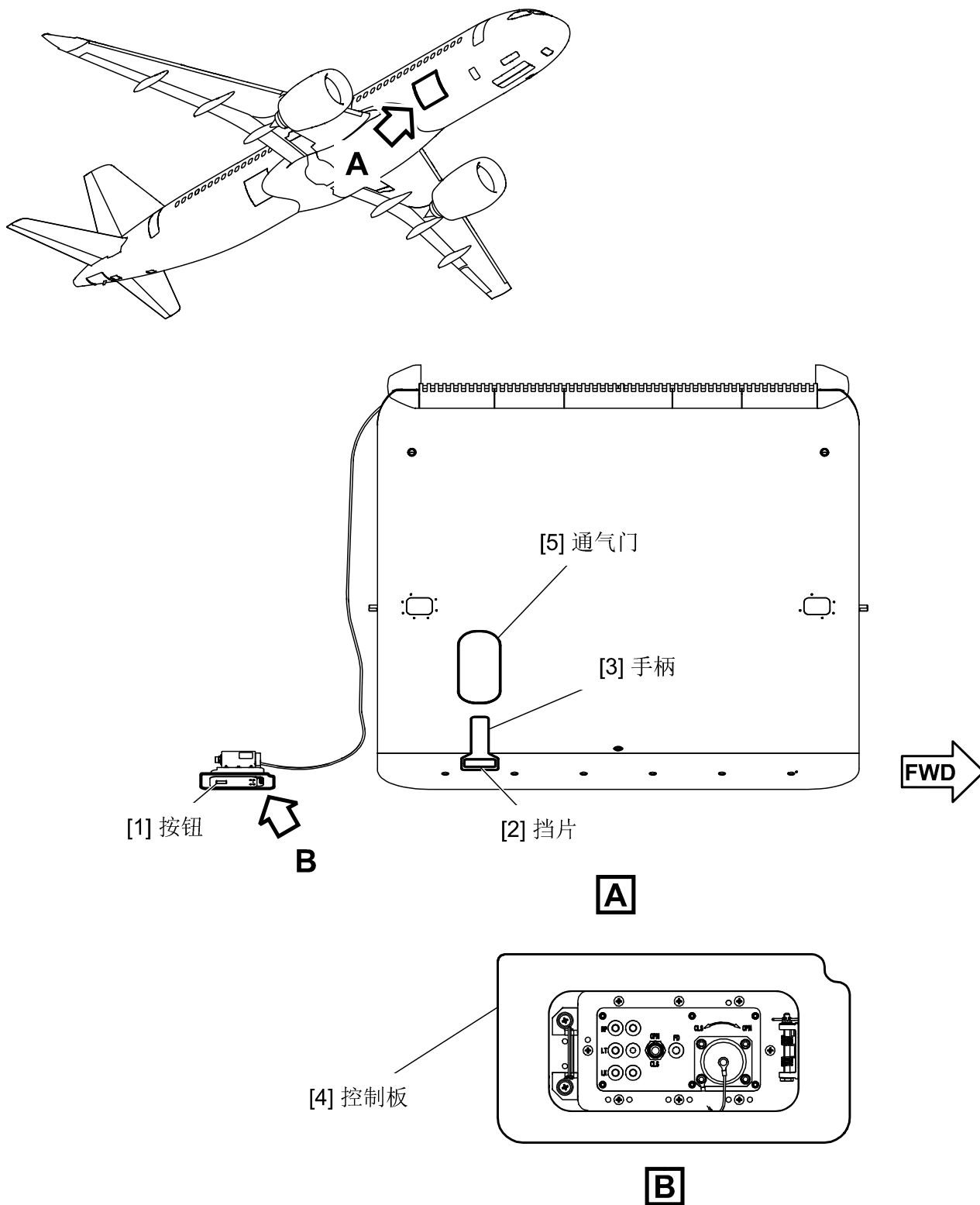
图 1 货舱门关闭(共1张 第1张)
