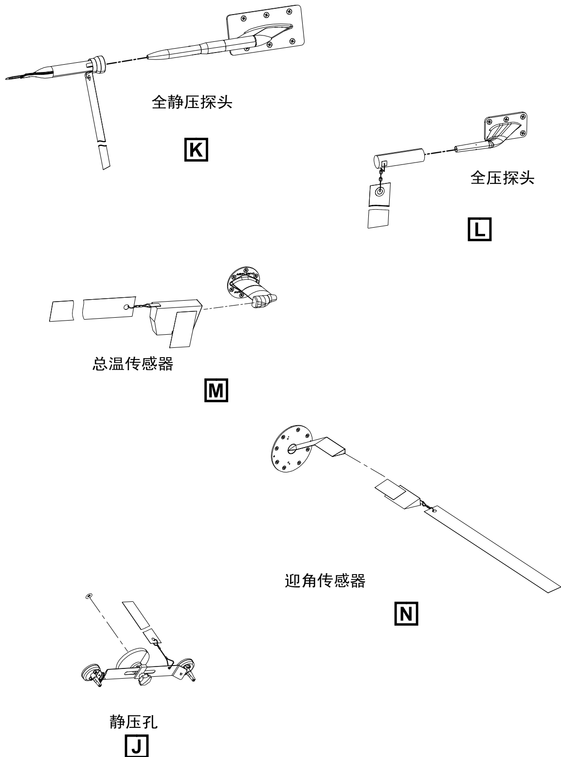
图 1 飞机保护装置-拆卸程序(共10张 第5张)
