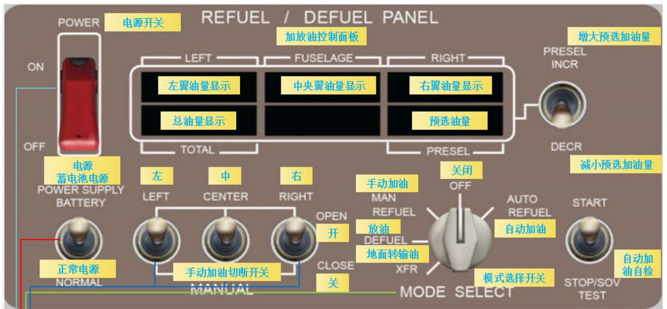
图 1 加油抽油控制面板(共1张 第1张)
