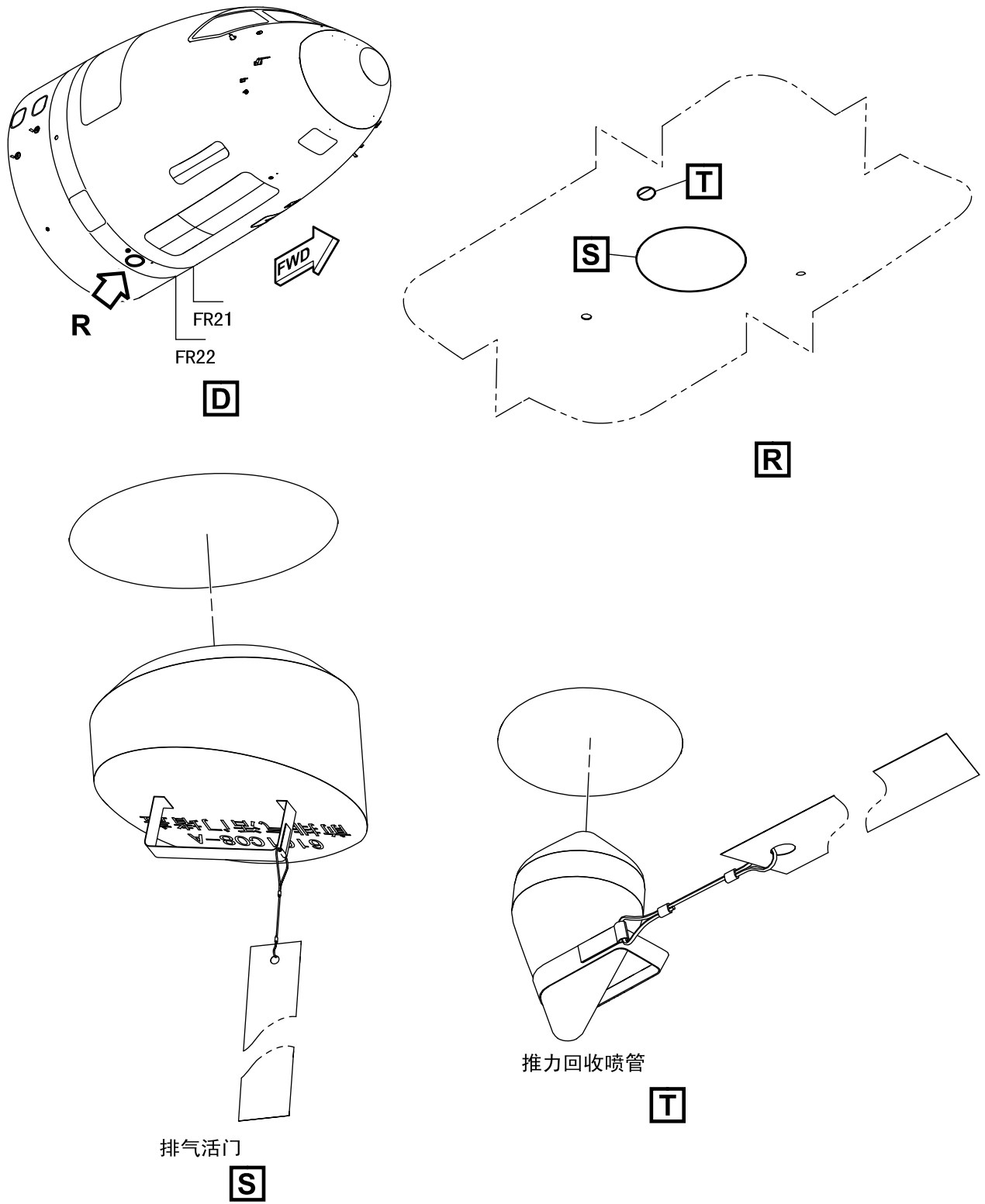
图 1 飞机保护装置-拆卸程序(共10张 第4张)
