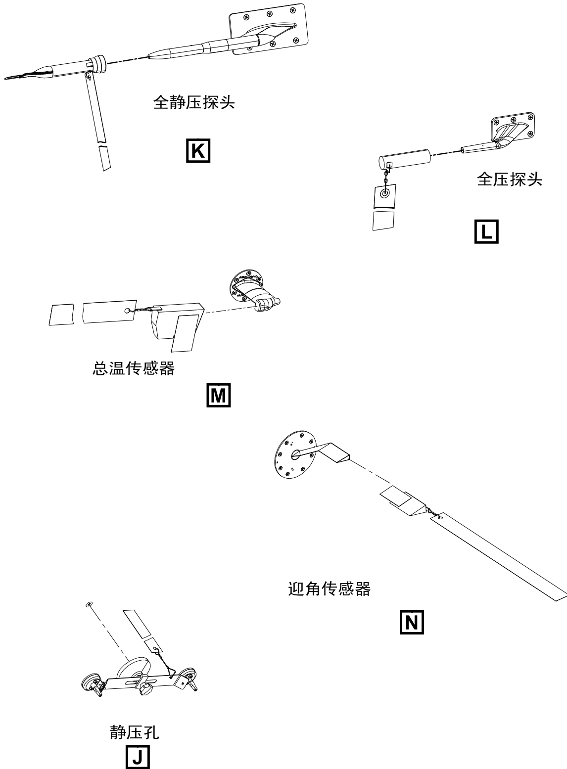
图 1 飞机保护装置-安装程序(共10张 第5张)
