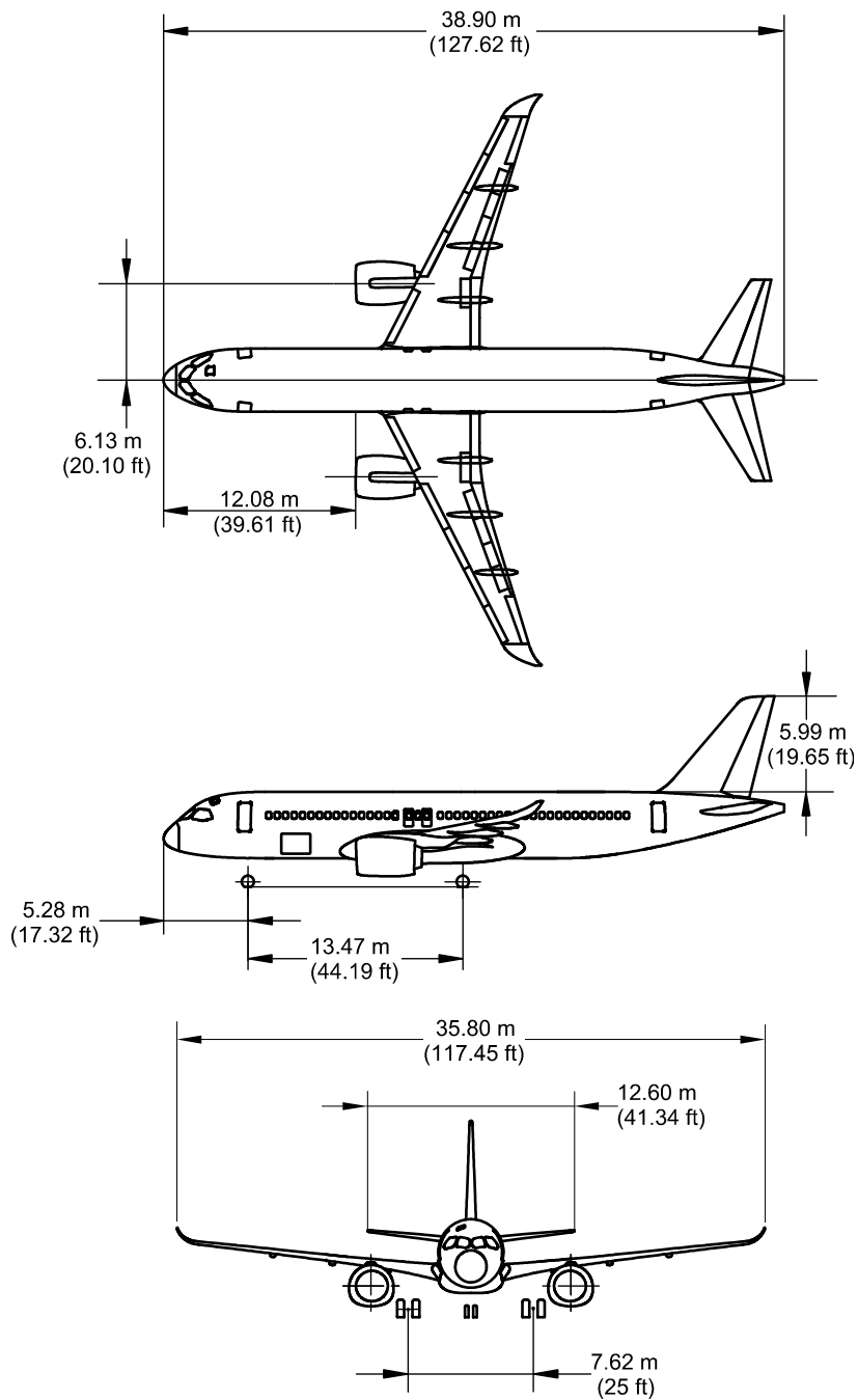
图 1 总体尺寸(共1张 第1张)
