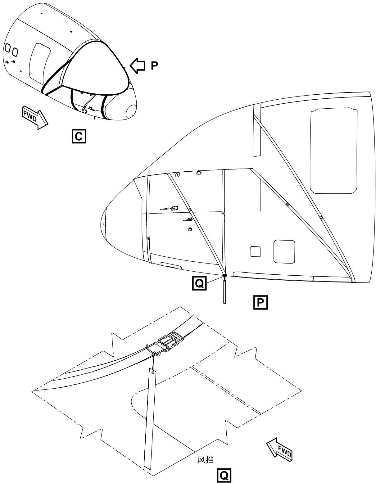
图 1 飞机保护装置-拆卸程序(共10张 第3张)
