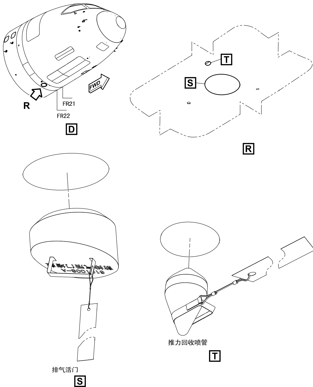
图 1 飞机保护装置-安装程序(共10张 第4张)
