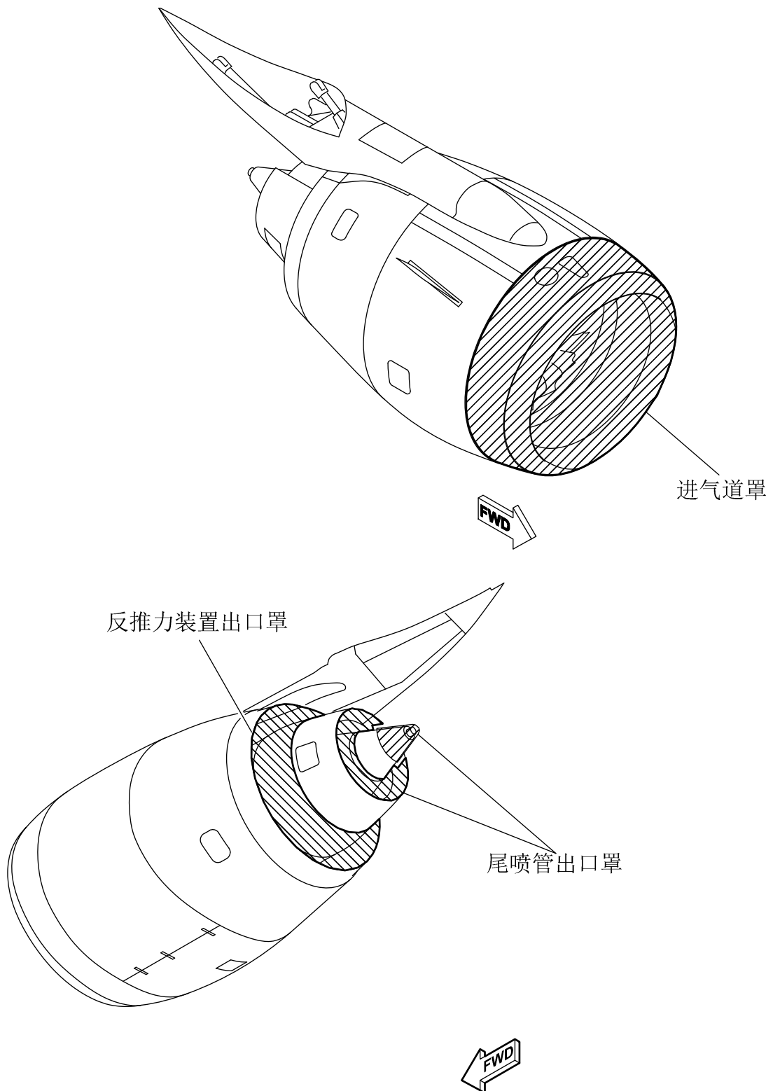
图 1 飞机保护装置-安装程序(共10张 第10张)
