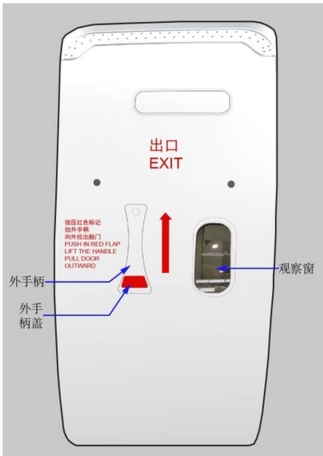
图 1 登机门外部关闭(共1张 第1张)
