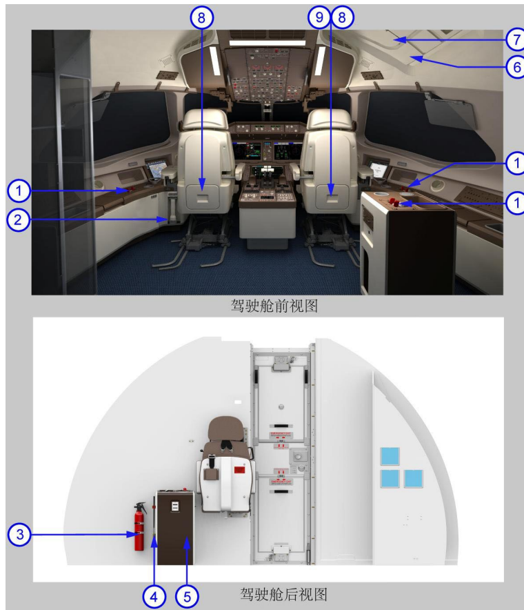
图 1 驾驶舱应急设备(共1张 第1张)
