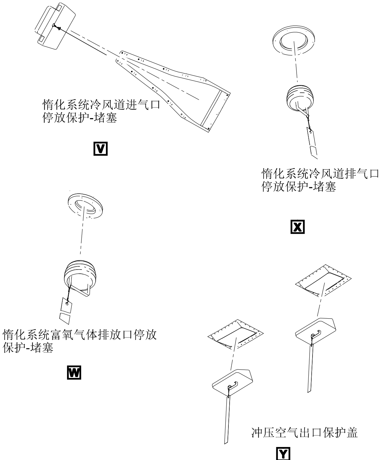
图 1 飞机保护装置-拆卸程序(共10张 第7张)
