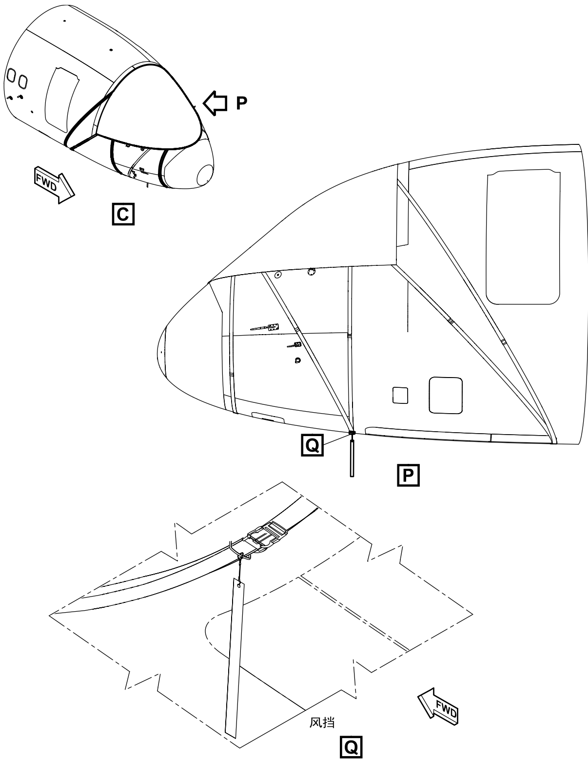
图 1 飞机保护装置-安装程序(共10张 第3张)
