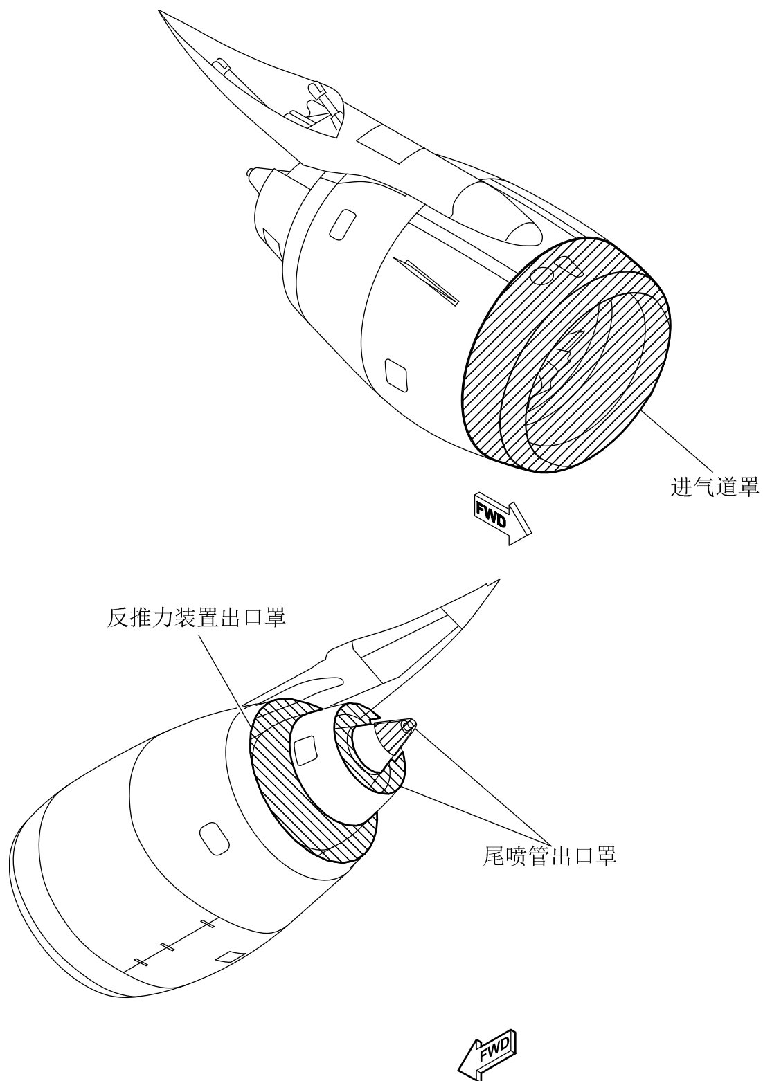
图 1 飞机保护装置-拆卸程序(共10张 第10张)
