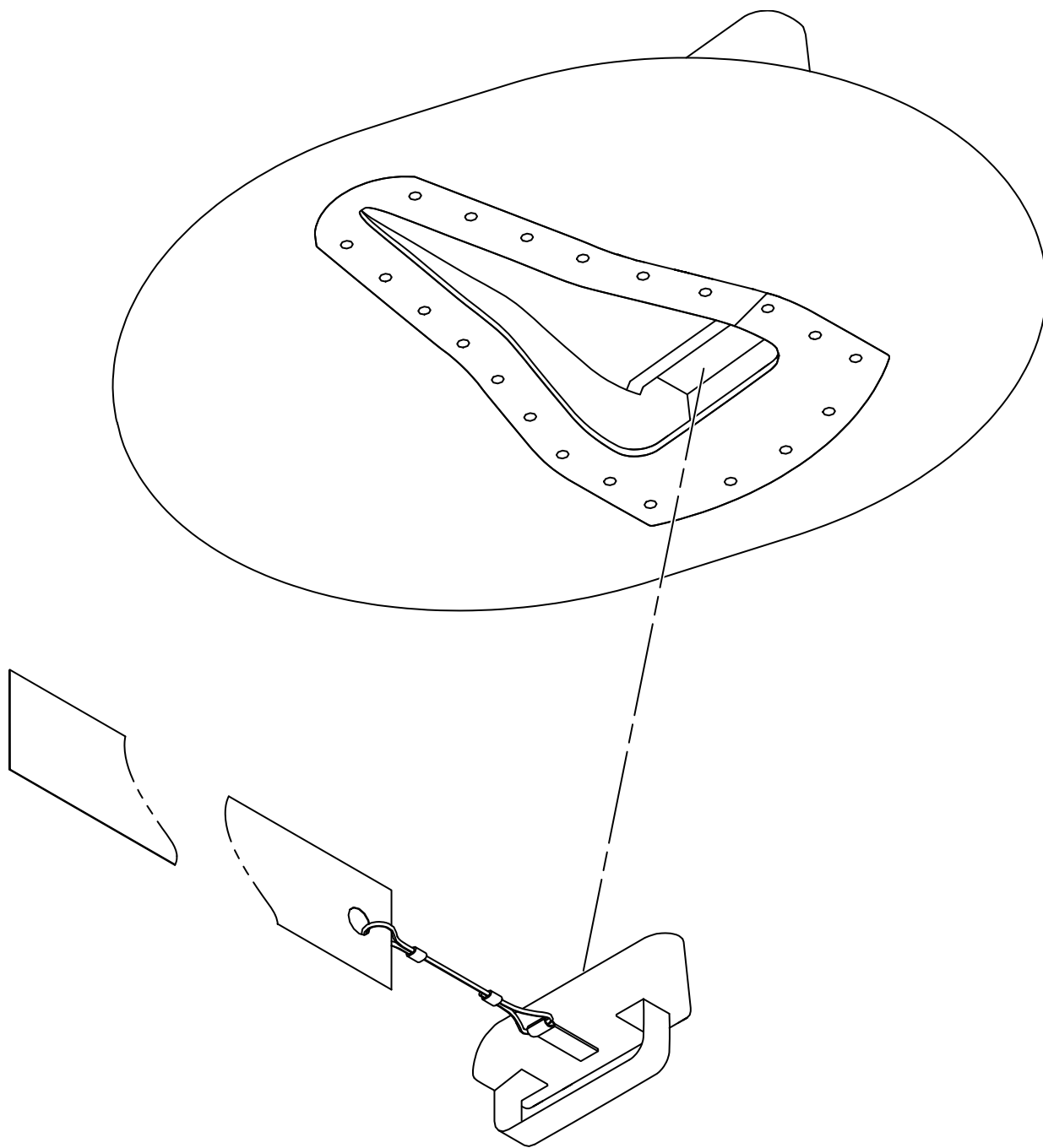
燃油箱NACA通气口
