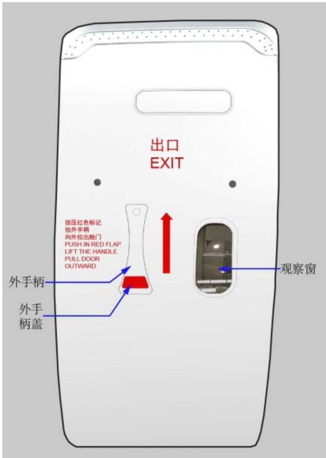
图 1 登机门外部打开(共1张 第1张)
