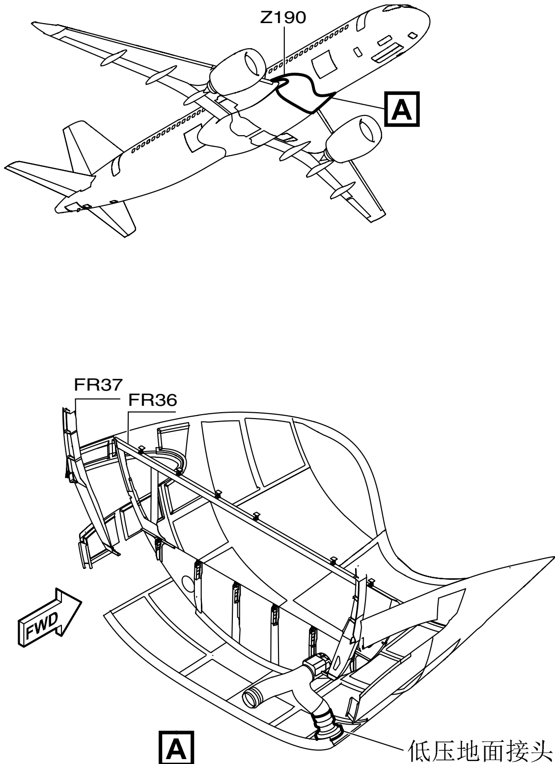
图 1 外部接头(共1张 第1张)
